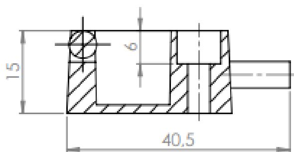
ŘEZ A-A
